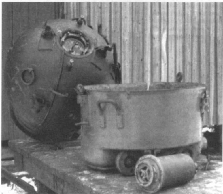
Мина МАВ-1, вытравленная финнами
