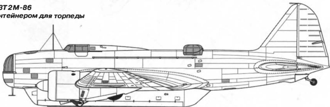
ДБ-3ТП 2М-86 с торпедой 45-36-АН
