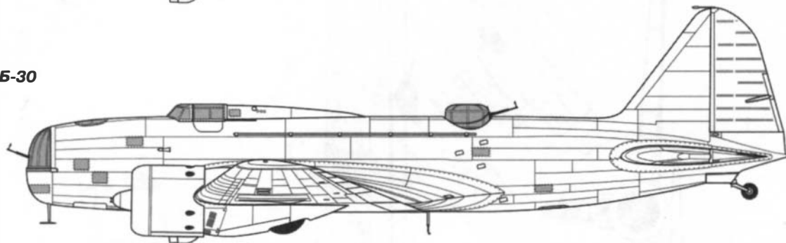
ДБ-3 2М-85 выпуска завода №39 с радиостанцией «Луч»
