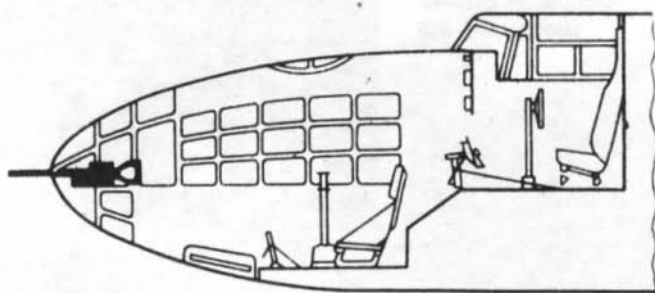
Компоновка носовой части самолетов модификаций Б (слева) и Ф (справа)
