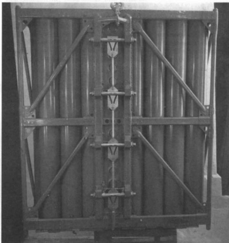
Ампульная кассета АК-2У
