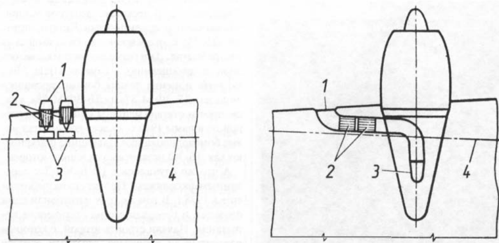
Схемы размещения маслорадиаторов на опытном и первых серийных ДБ-3Ф (слева) и на последующих сериях (справа): 1 — воздухозаборник; 2 — маслорадиаторы; 3 — выход охлаждающего воздуха; 4 — ось переднего лонжерона крыла
