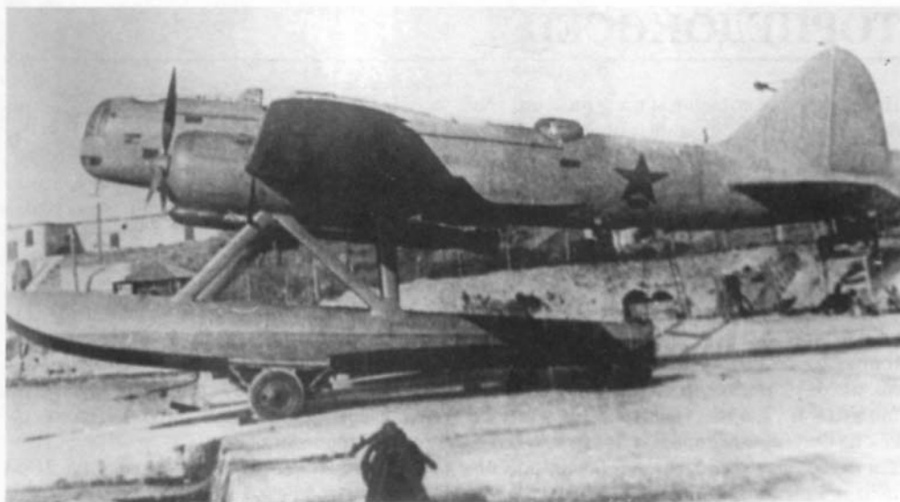
ДБ-3ПТ с подвешенной торпедой 45-36АН на испытаниях в Севастополе, октябрь 1938 г.
